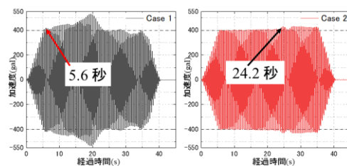
Fig. 7 加速度の変化 (a1, Case1, Case2) Acceleration trend
